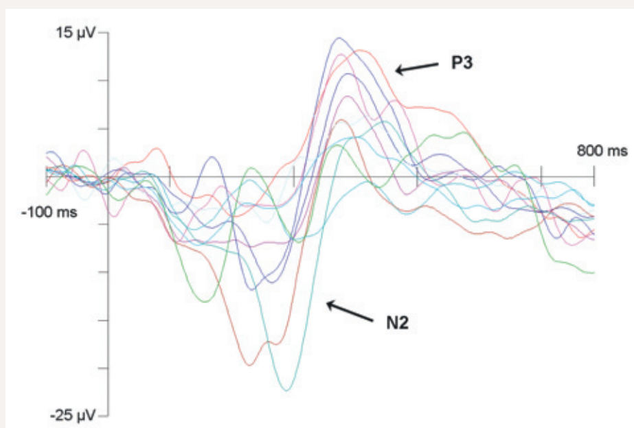
11 friske personers hjerneaktivitet knyttet til stavelsen /ta/ som ble aktivt oppdaget blant standardstavelsen /ba/ (elektrode: Pz). De hendelsesrelaterte potensialene N2 og P3 er markert. Basert på data fra Becker & Reinvang [9]
