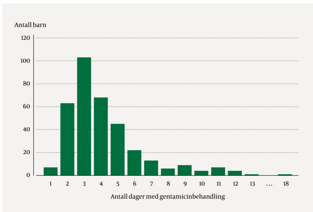
Figur 1 Behandlingsvarighet for 353 gentamicinbehandlingsepisoder ved St. Olavs hospital og Universitetssykehuset Nord-Norge der det også ble tatt s-gentamicin-o-prøve. Barn i alderen 1 måned til 17 år.
