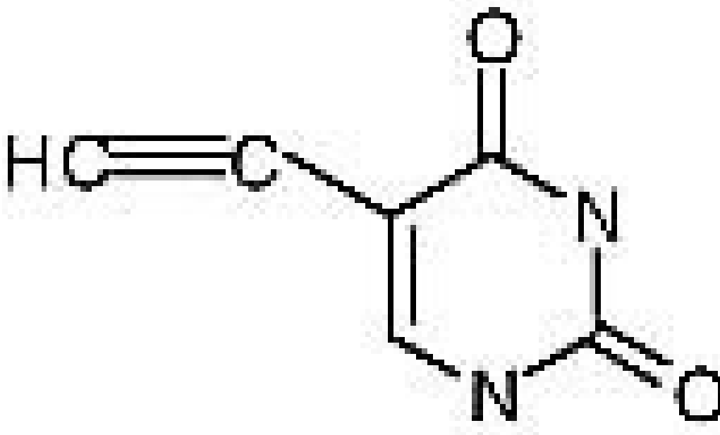
Figur 5 Kjemisk struktur for eniluracil
