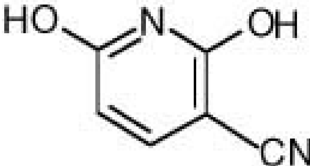
Figur 7 Kjemisk struktur for CNDP (3-cyano-2,6-dihydroksypyrimidin)
